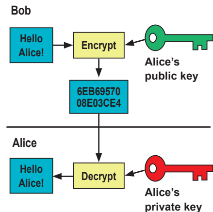
Εικόνα 6.1 Ασύμμετρη Κρυπτογράφηση
