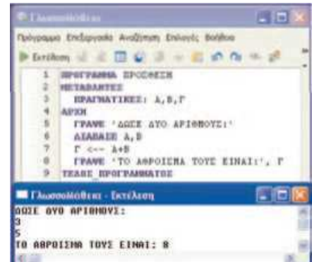
Εικόνα 1.4. Ο κώδικας για την άθροιση δύο αριθμών στο προγραμματιστικό περιβάλλον Γλωσσολάβητα.
